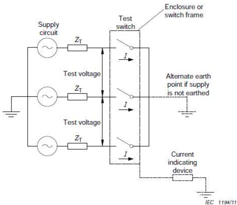
شکل ۶: مدار آزمون جریان وصل اتصال کوتاه
